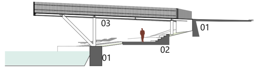
CORTE EE esc. 1:250
